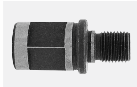
Артикул 1420019121 Переходник Weldon 19 на 1/2 20UNF
